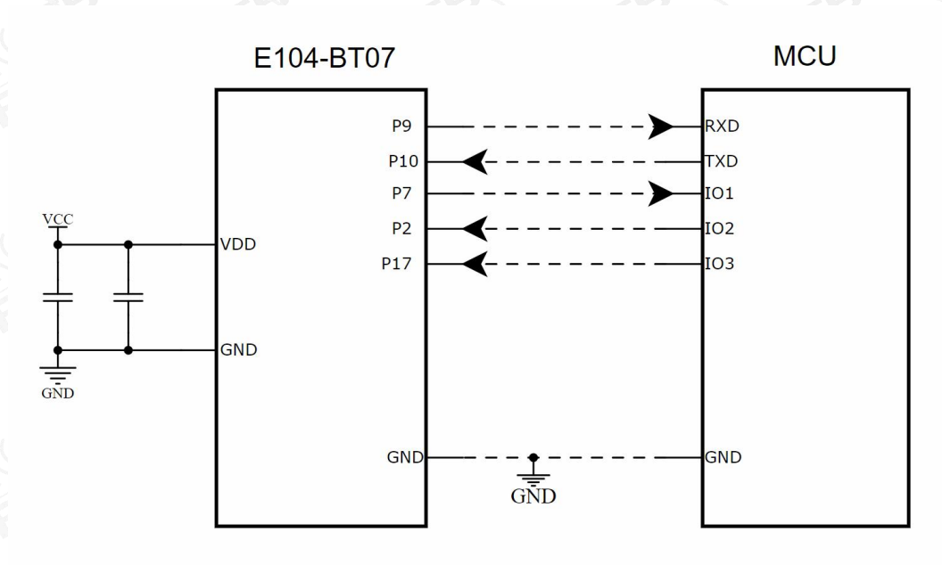
Figure 4-1 E104-BT07 Circuit
