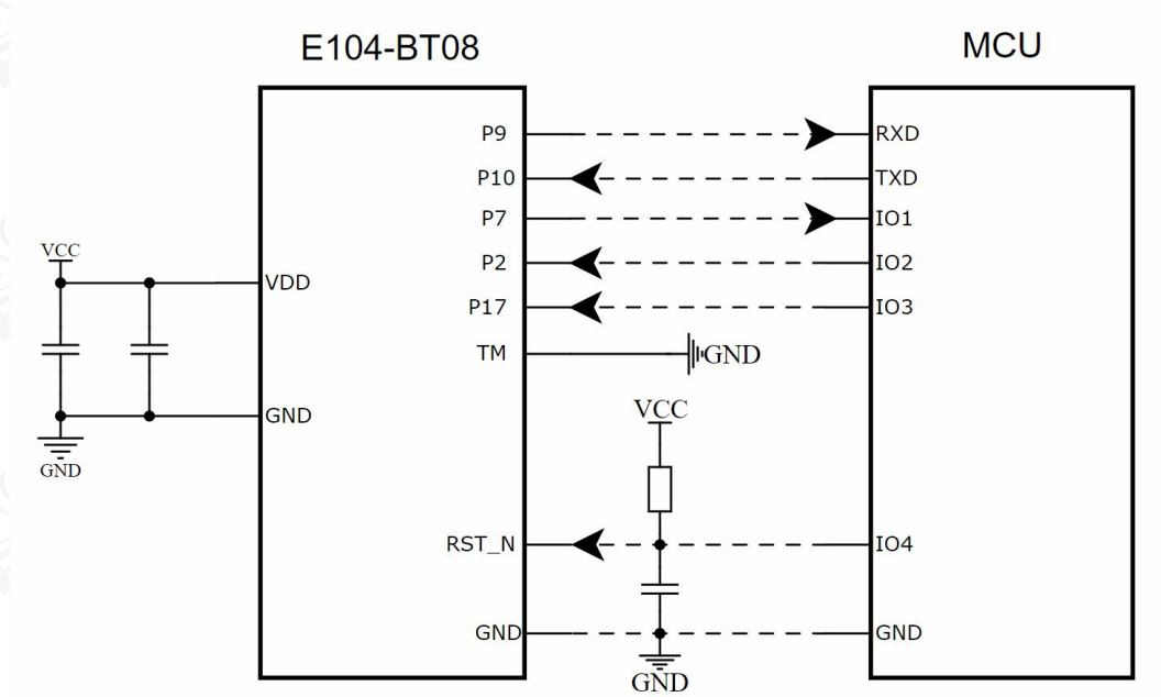
Figure 4-2 E104-BT08 Circuit
